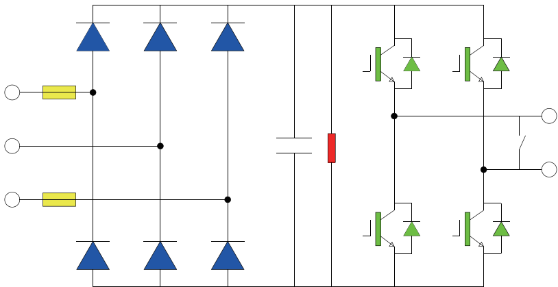
图2-5 功率单元原理图
